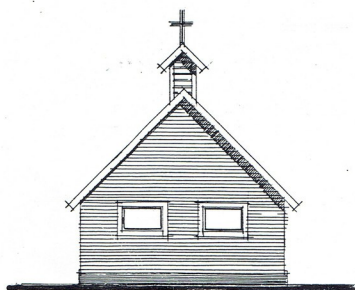
Elewacja południowo zachodnia
